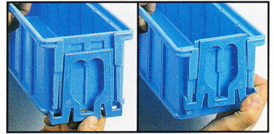
Einfügen des Handgriffs F PK 6051 00 04 - F PK 6651 00 04
